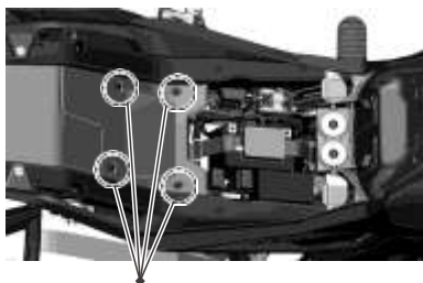
Kołki dystansujące
